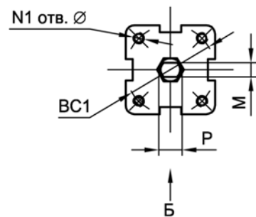
А-А (1:1, фиксатор не показан)
