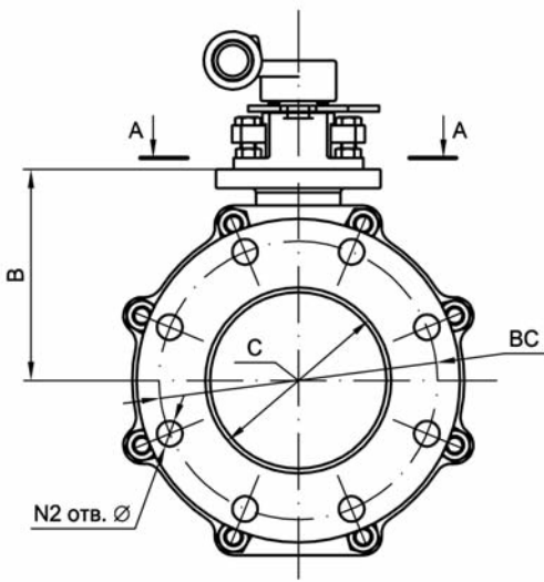
Б (1:2, фиксатор не показан)
