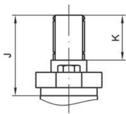
А-А (1:2, фиксатор не показан)
